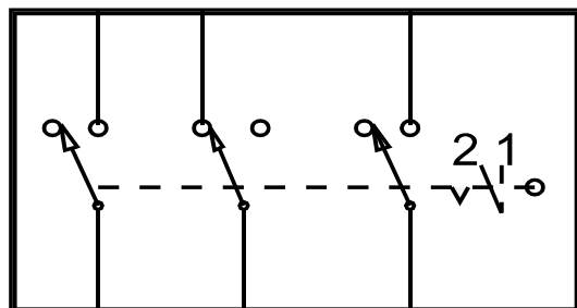
多路开关
